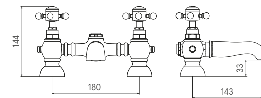
BATH FILLER
