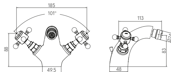
BIDET MIXER TAP
